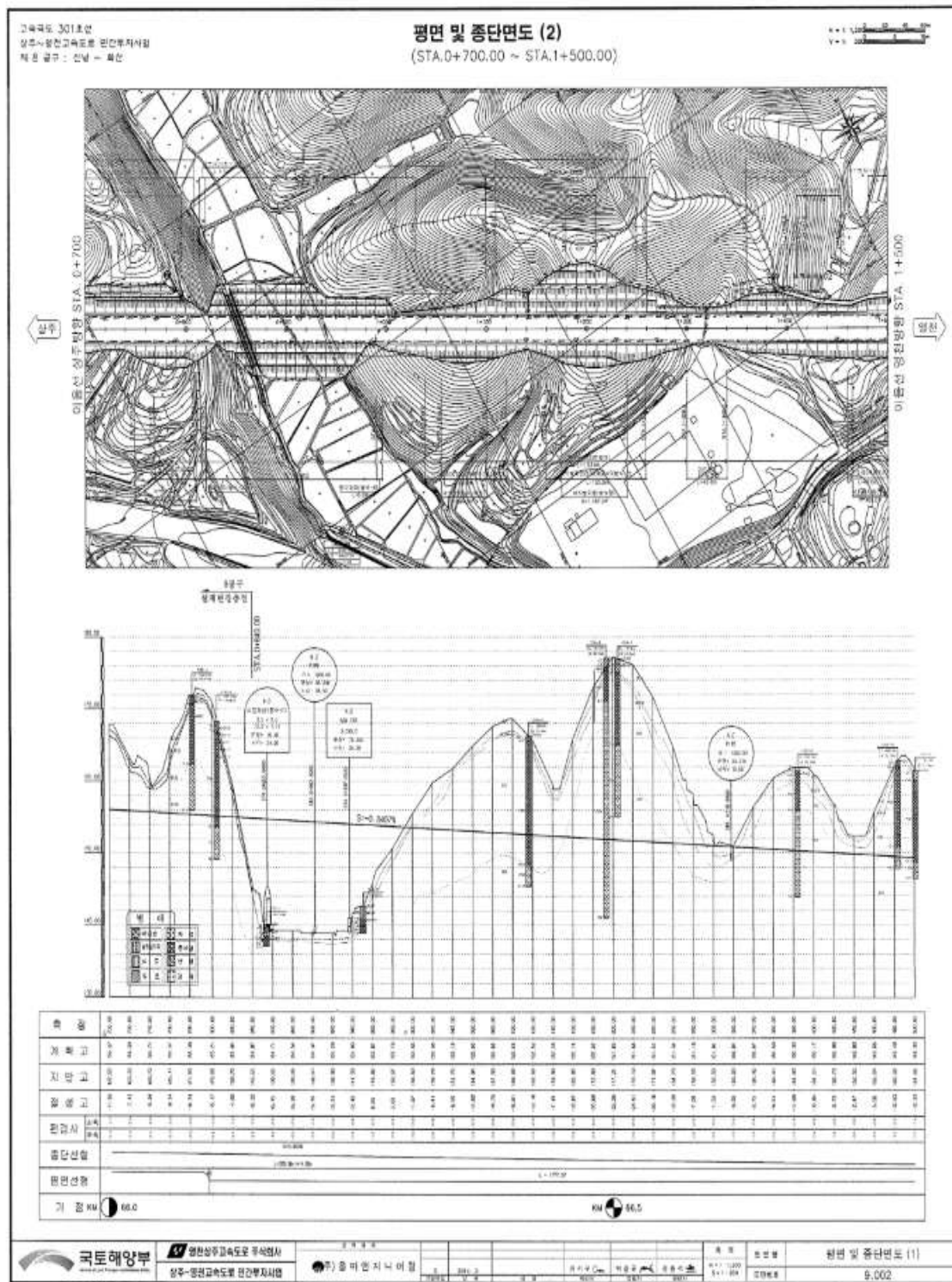
【그림 44.3】 평면도
