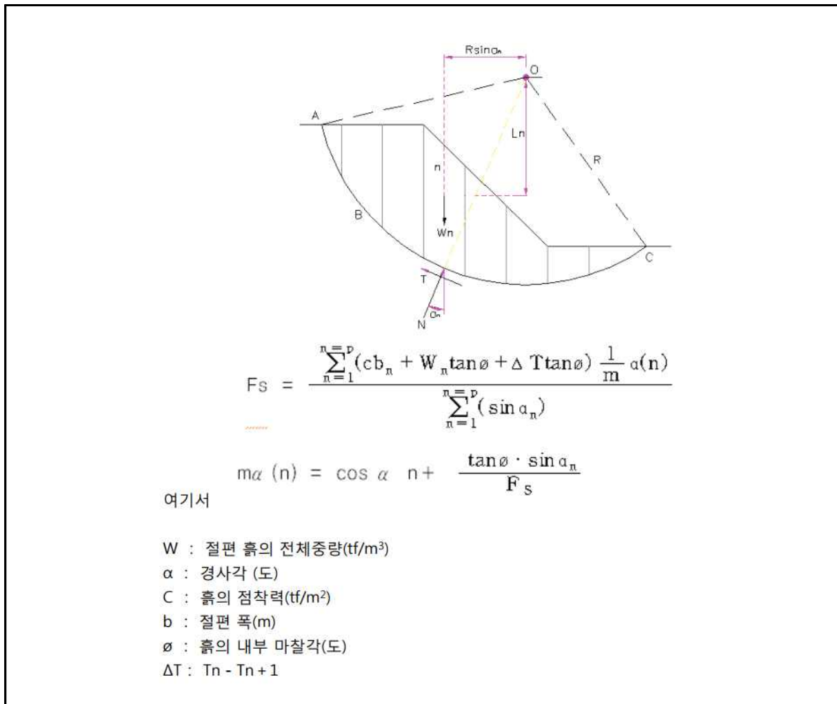
【그림 44.7】 Bishop의 안전율 계산식
