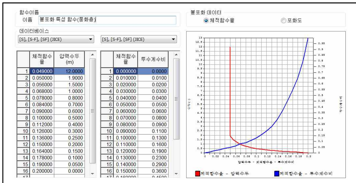
【그림 44.15】 압력수두-채적함수율(포화도)-투수계수비 함수
