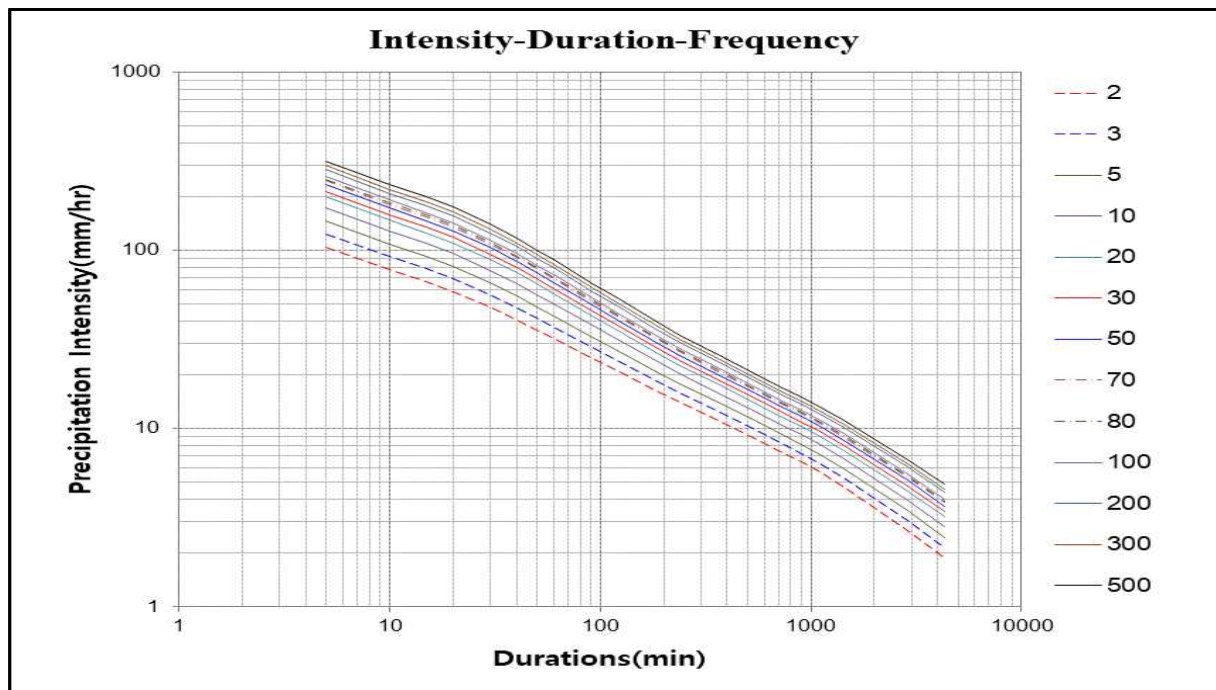
【그림 44.9】 영천지역 IDF곡선
